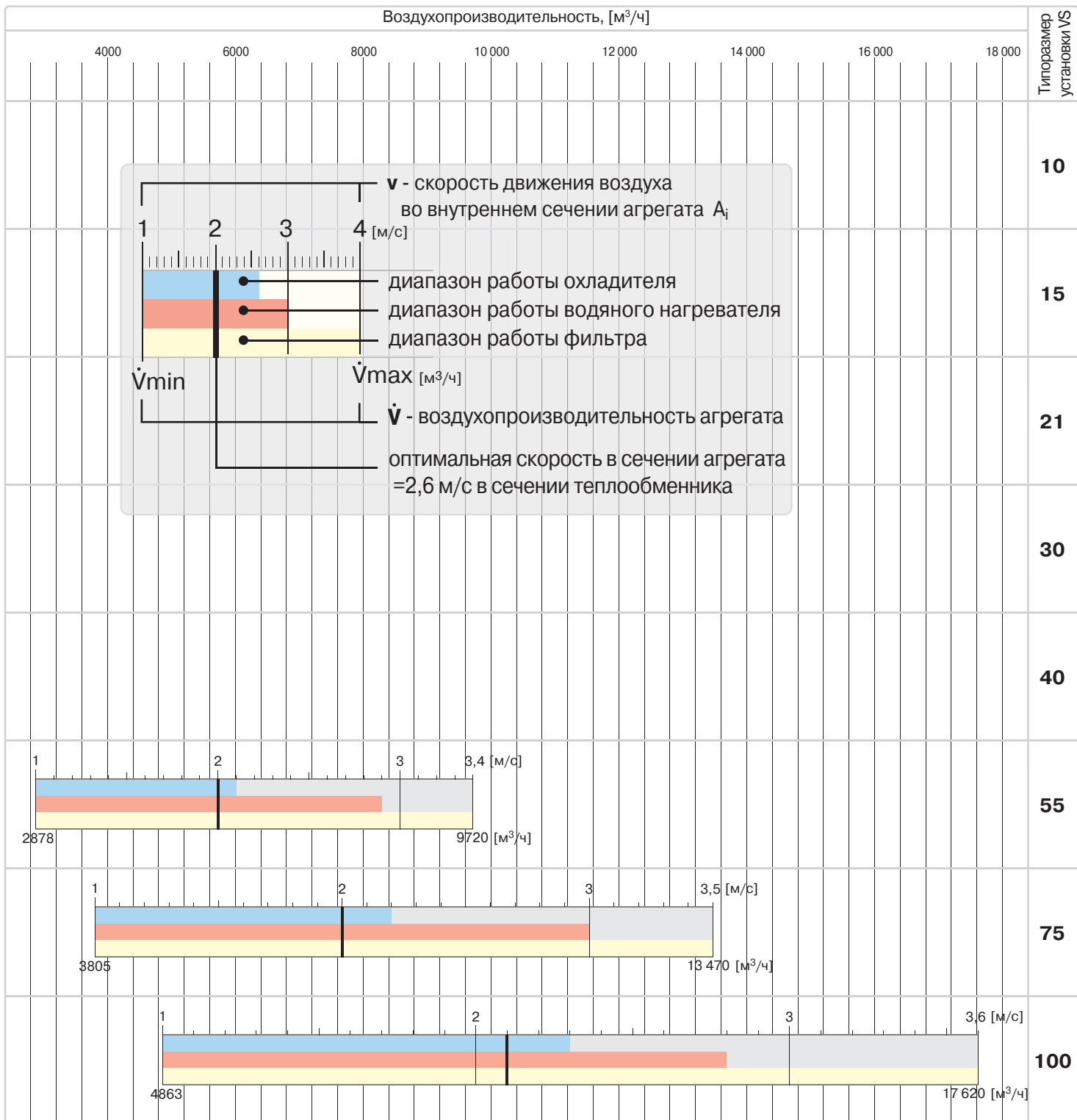
Максимальные скорости воздуха v_{max} [м/с]
